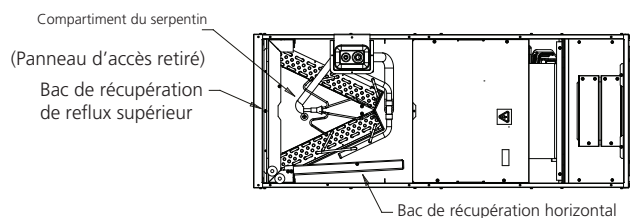
Fig. 1 – Représentation de l'appareil intérieur
