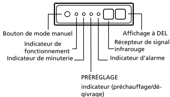
Fig. 2 – Panneau d'affichage du récepteur infrarouge (IR)
