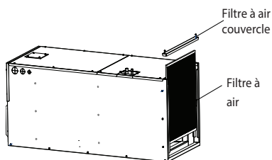
Fig. 4 – Retirez le couvercle du filtre à air
