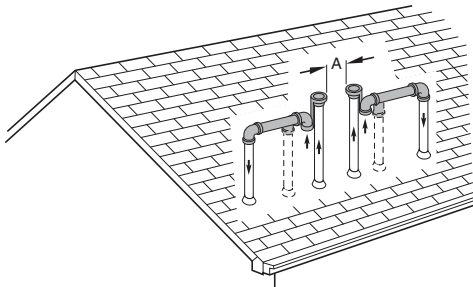
Fig. 46 – Ventilación de tubería y de combustión
