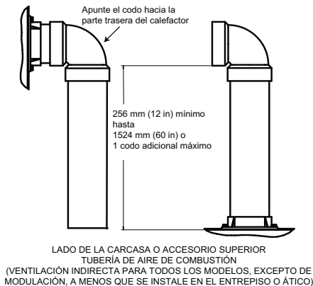
Fig. 45 – Accesorio de tubería de aire de combustión
