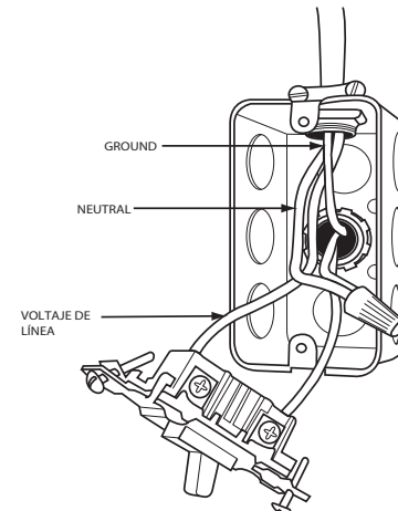
Fig. 35 – Caja eléctrica externa
