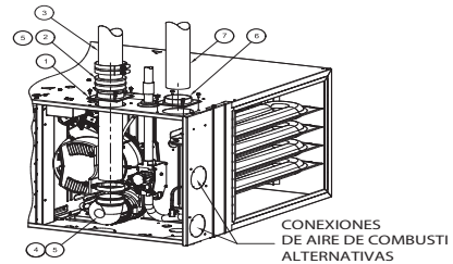
CONFIGURACIÓN DE VENTILACIÓN VERTICAL DERECHA HORIZONTAL
