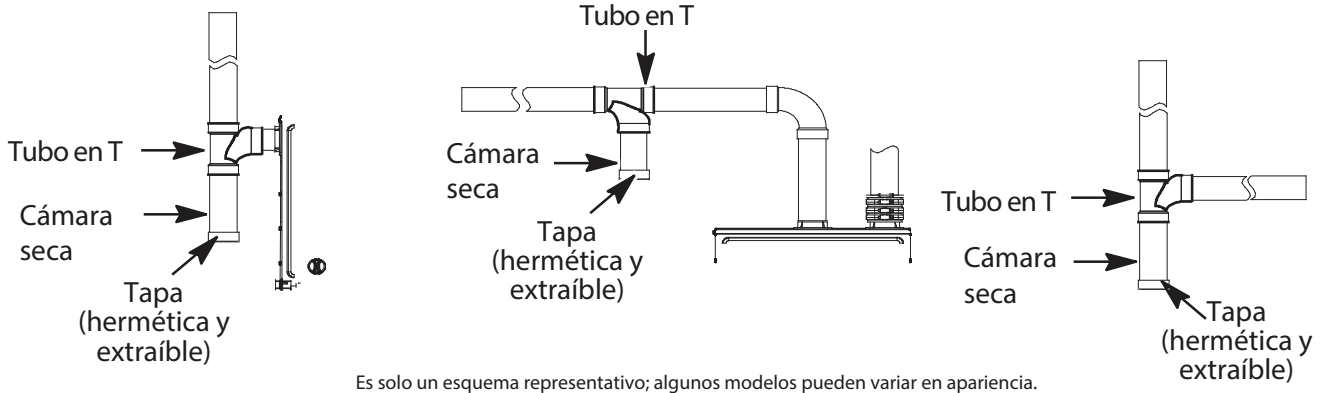
Fig. 51 – Trampa de humedad de admisión de aire de combustión recomendada
