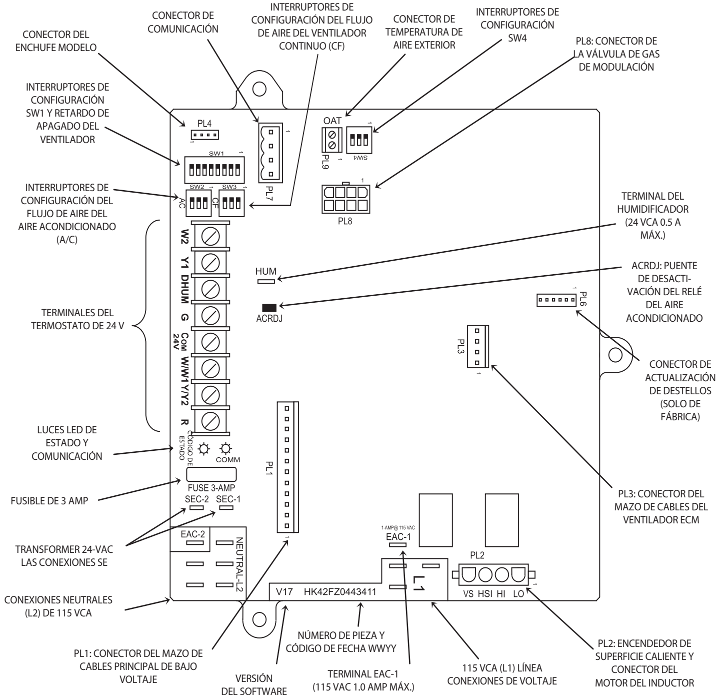
Fig. 37 – Ejemplo de control del calefactor variable
