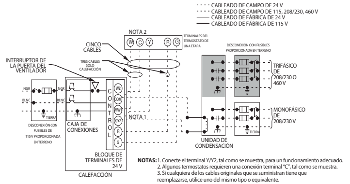
Fig. 32 – Diagrama eléctrico típico in situ
