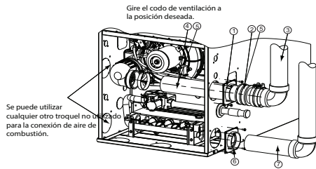
CONFIGURACIÓN CON FLUJO DESCENDENTE HACIA LA DERECHA
