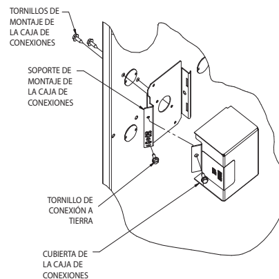
Fig. 34 – Instalación de la caja de conexiones (cuando se usa) La apariencia puede variar
