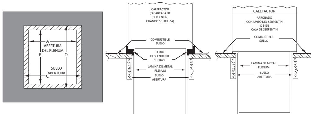
Fig. 24 – Instalación sobre piso combustible
