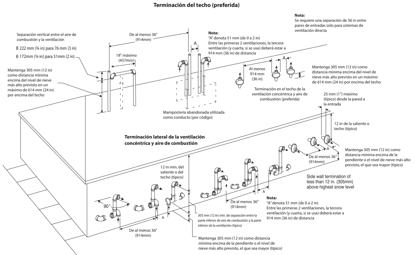
Fig. 40 – Terminación de aire de combustión y de ventilación para sistemas de ventilación directa (2 tuberías)
