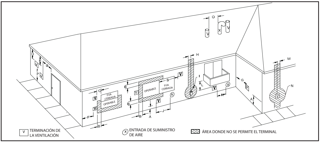
Fig. 42 – Distancia de la terminación de ventilación directa
