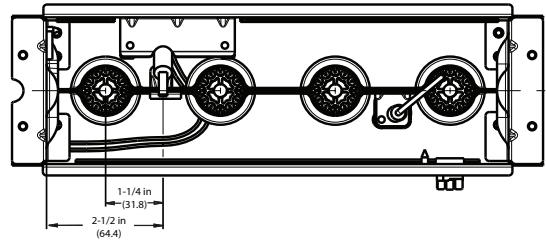
Fig. 70 – Posición del encendedor: vista superior
