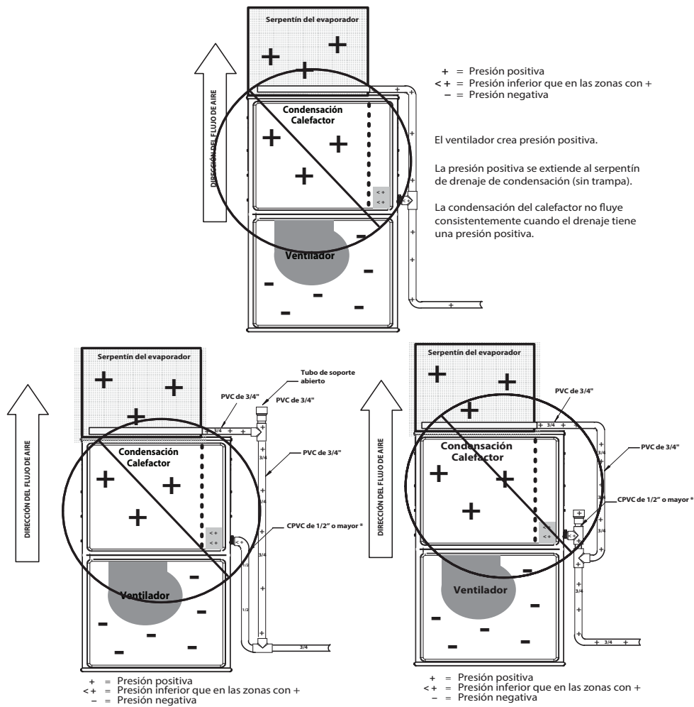
Fig. 12 – Ejemplo de conexión del drenaje in situ (no permitido)
