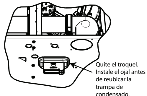
Fig. 17 – Arandela para la trampa de drenaje horizontal
