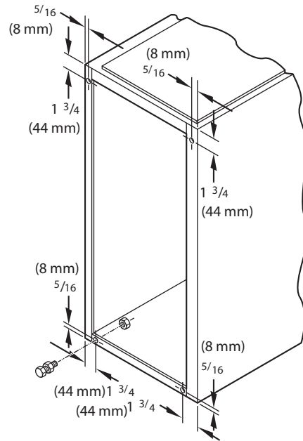
Fig. 28 – Patas niveladoras
