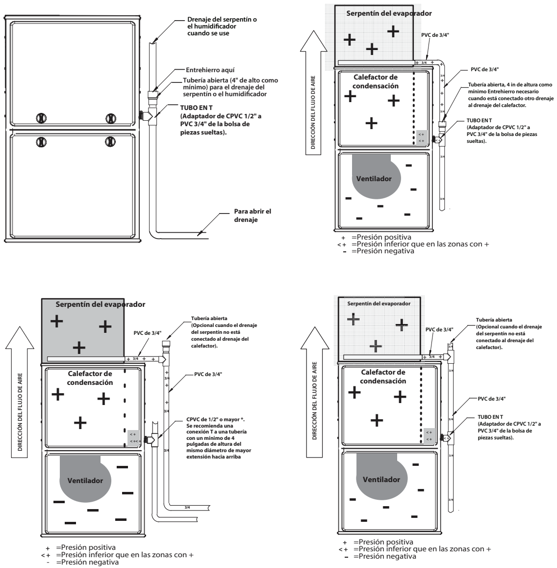
Fig. 11 – Ejemplo de conexión del drenaje in situ
