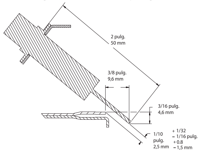
Fig. 71 – Posición del encendedor: vista lateral
