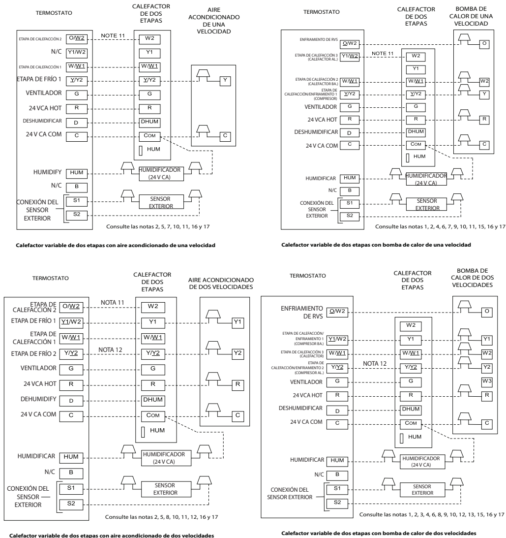
Calefactor variable de dos etapas con aire acondicionado de dos velocidades
