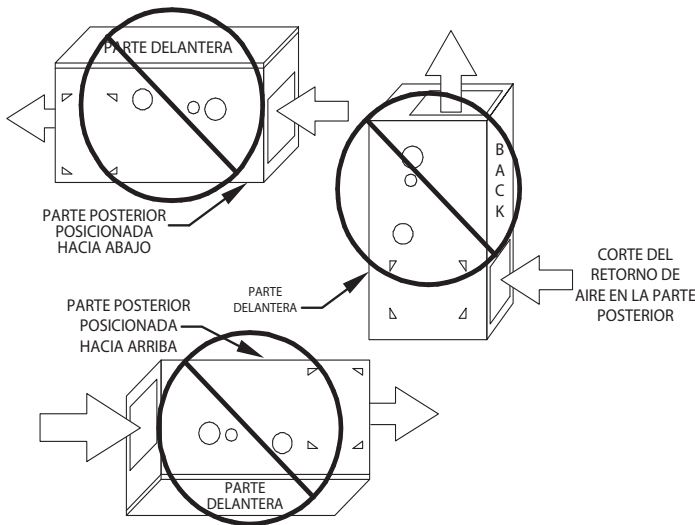
Fig. 4 – Instalaciones prohibidas
