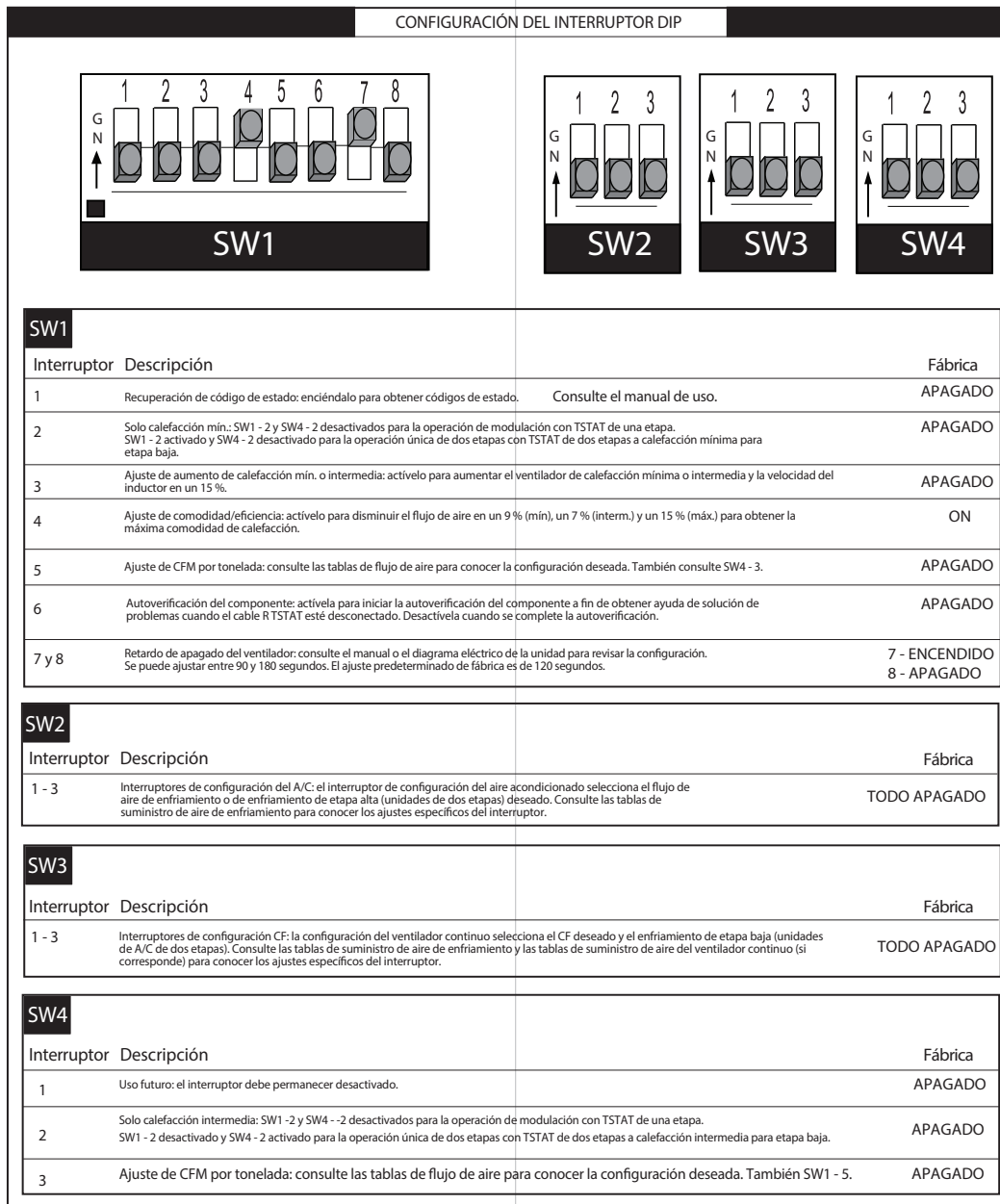
Fig. 60 – Interruptores de configuración y descripción del calefactor
