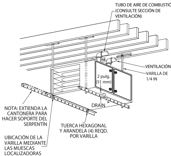
Fig. 26 – Plataforma de trabajo para instalaciones en áticos
