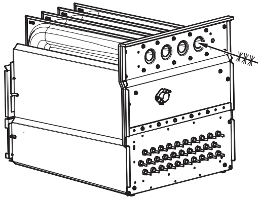
Fig. 72 – Limpieza de la celda del intercambiador de calor A11273
