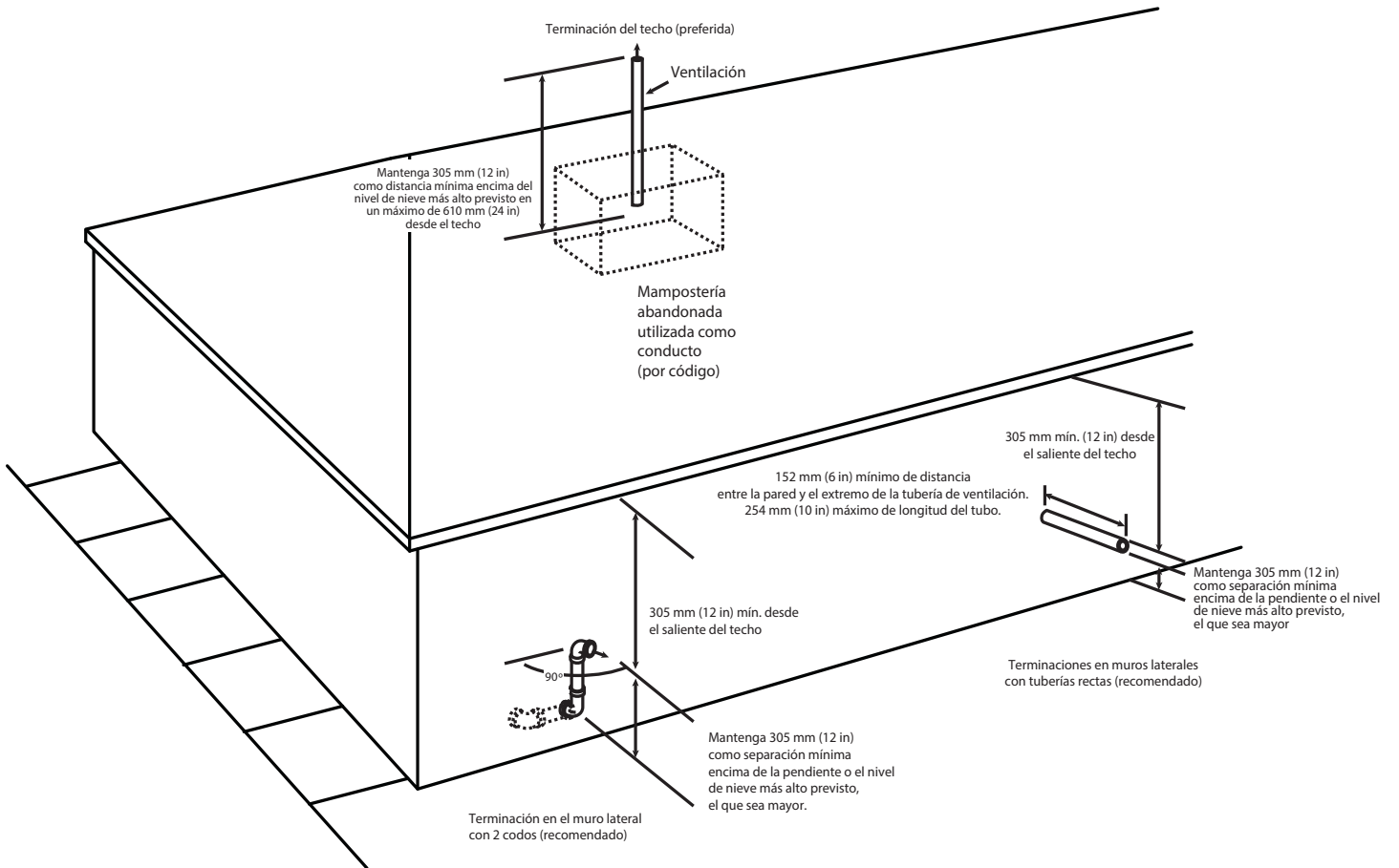
Fig. 41 – Terminación de la tubería de ventilación para sistemas de ventilación indirecta y de aire de combustión ventilado
