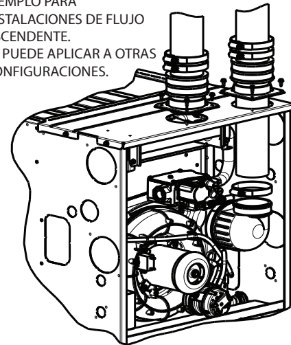
Fig. 50 – Ejemplo de conexión de la tubería de aire de admisión para sistemas de ventilación de polipropileno
