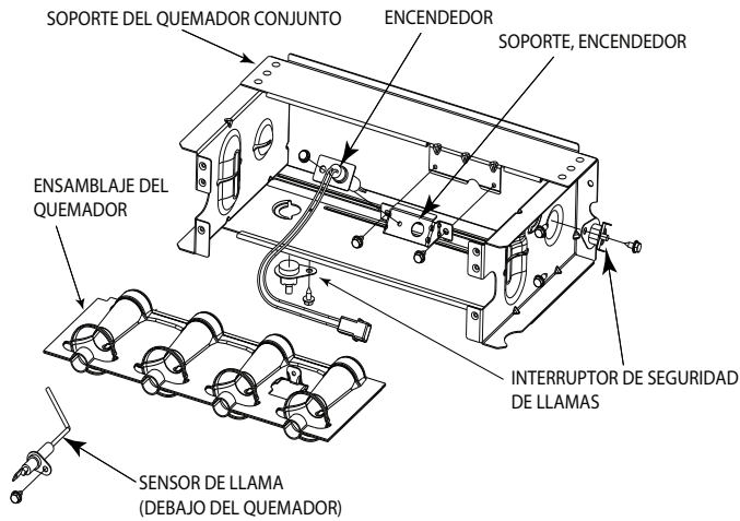
Fig. 69 – Conjunto del quemador
