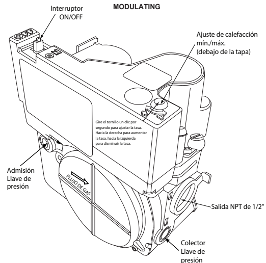
Fig. 64 – Válvula de gas sin puertos de presión de torre A10496
