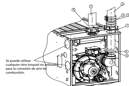
VENTILACIÓN VERTICAL CON FLUJO ASCENDENTE
