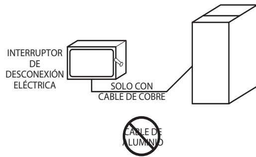
Fig. 33 – Caja eléctrica externa no incluida en la carcasa del calefactor
