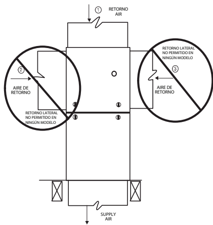
Fig. 21 – Configuraciones de aire de retorno de flujo descendente and Restrictions A11037
