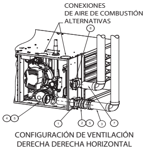
CONFIGURACIÓN DE VENTILACIÓN DERECHA HORIZONTAL A LA DERECHA
