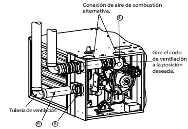
CONFIGURACIÓN DE VENTILACIÓN IZQUIERDA IZQUIERDA HORIZONTAL
