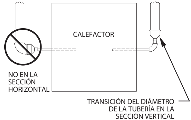
Fig. 48 – Ubicación de la transición del diámetro de las tuberías de aire de combustión y ventilación y configuración del codo
