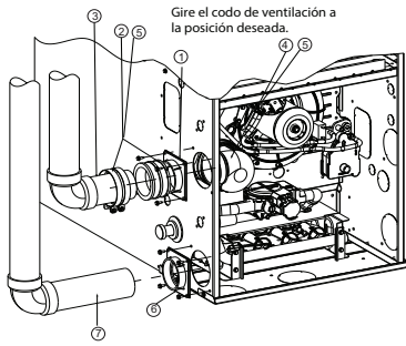
CONFIGURACIÓN CON FLUJO DESCENDENTE HACIA LA IZQUIERDA
