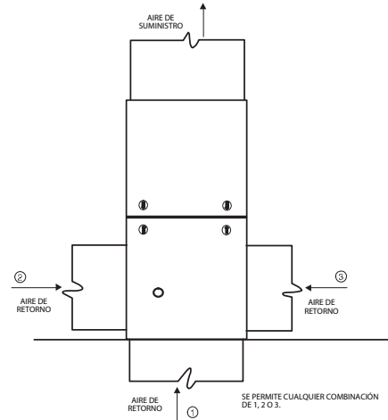
Fig. 20 – Configuraciones y restricciones de aire de retorno de flujo ascendente
