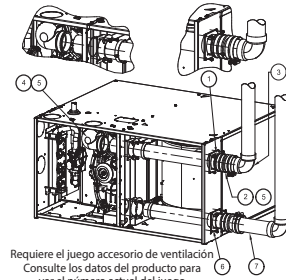
CONFIGURACIÓN DE VENTILACIÓN DERECHA IZQUIERDA HORIZONTAL
