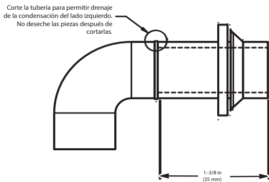
Fig. 16 – Modificación del codo de goma de drenaje
