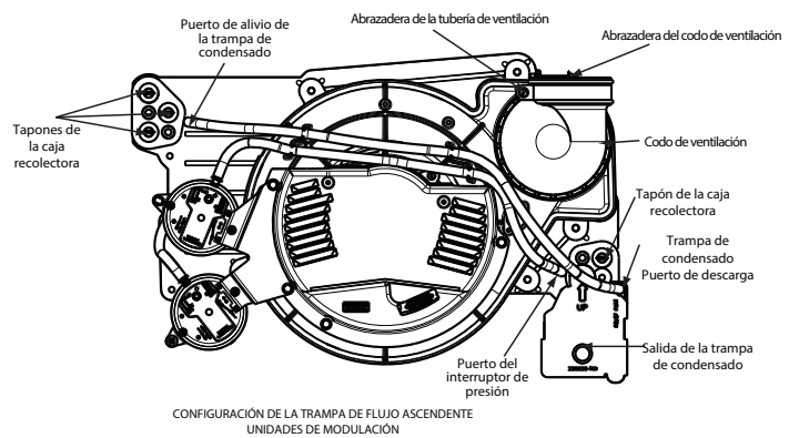
Fig. 7 – Configuración de la trampa de flujo ascendente (La apariencia puede variar)
