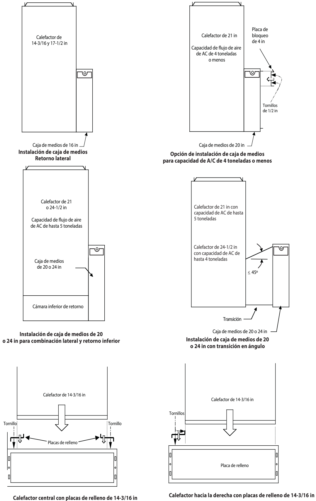
Fig. 25 – Filtro de medios
