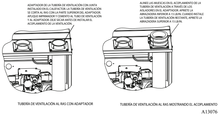
Fig. 59 – Tubería opcional de ventilación al ras con adaptador
