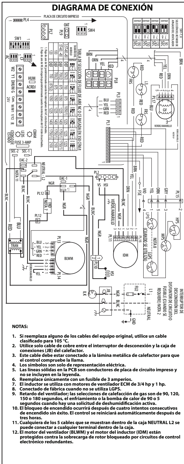
Fig. 74 – Diagrama eléctrico
