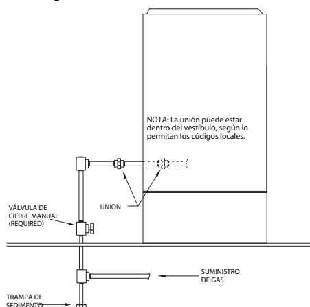
Fig. 31 – Disposición típica de las tuberías de gas
