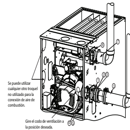
CONFIGURACIÓN CON FLUJO ASCENDENTE HACIA LA DERECHA
