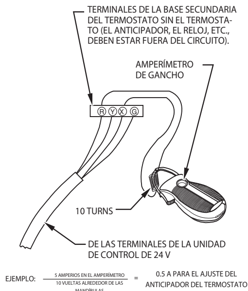
Fig. 66 – Verificación del amperaje con un amperímetro Ajuste el anticipador de calor del termostato.
