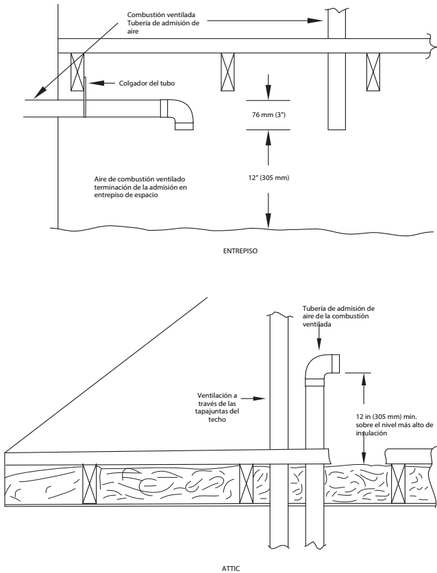
Fig. 47 – Terminaciones de ventilación para sistemas de aire de combustión ventilado
