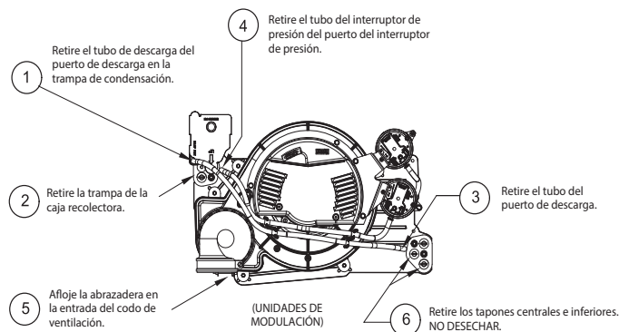
Configuración de fábrica no convertida Tal como se muestra en la orientación de flujo descendente
