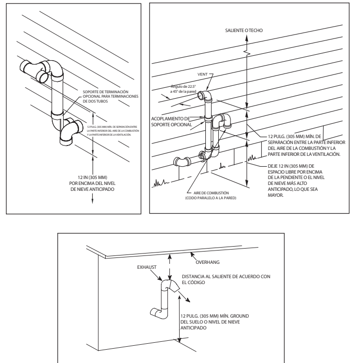
Fig. 49 – Terminación de ventilación en Alberta y Saskatchewan
