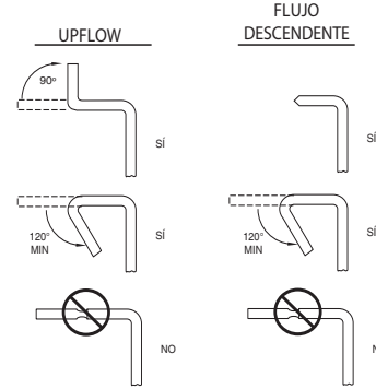
Fig. 19 – Bridas de conductos
