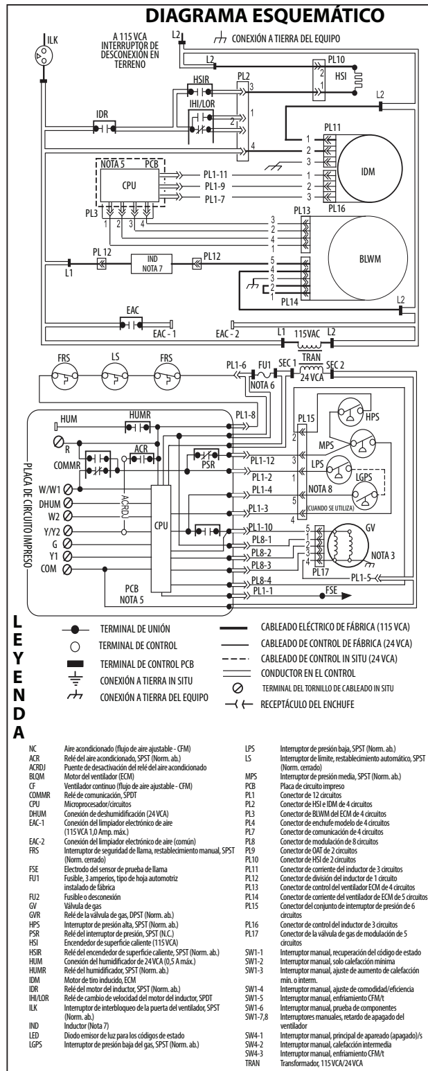
Fig. 74 – Diagrama eléctrico
