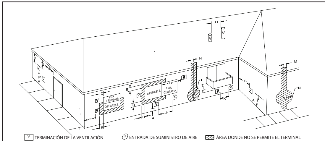
Fig. 43 – Distancias para las terminaciones de ventilación de aire de combustión ventilado y de ventilación indirecta
