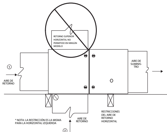
Fig. 22 – Configuraciones de aire de retorno horizontal and Restrictions A11038
