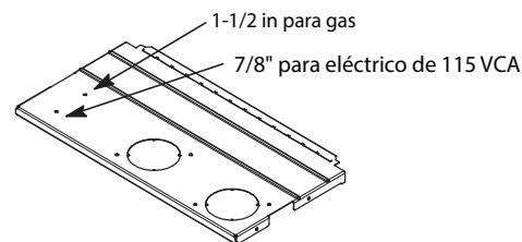
Fig. 30 – Entrada de gas y electricidad alternativa
