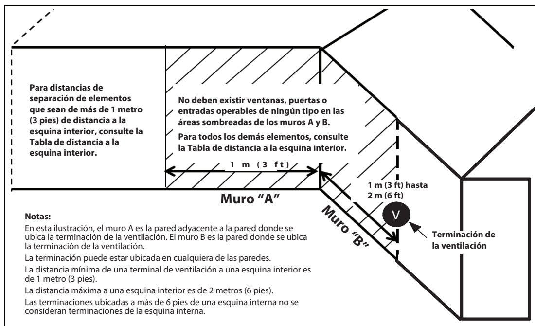
Fig. 44 – Terminación en esquina hacia dentro
