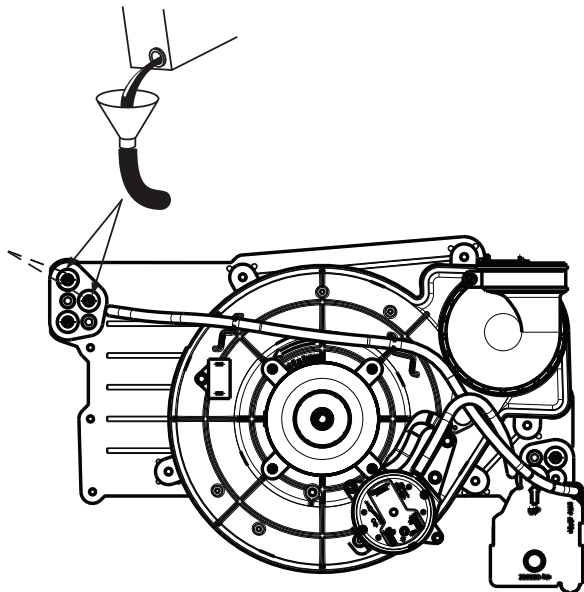
Fig. 61 – Cebado de la trampa de condensación (La apariencia puede variar)
