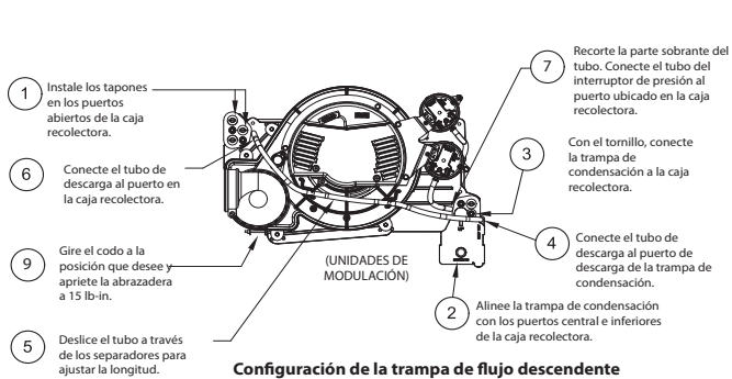
Configuración de la trampa de flujo descendente
