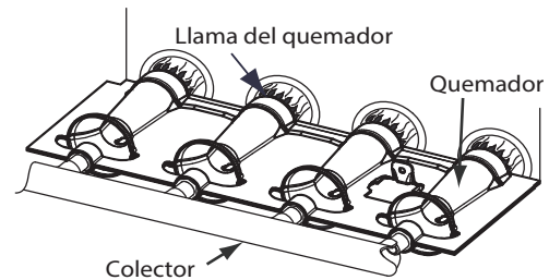
Fig. 65 – Llama del quemador
