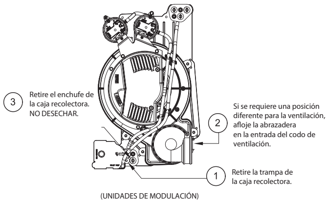
(UNIDADES DE MODULACIÓN) Configuración de fábrica no convertida de la trampa Tal como se muestra en la orientación horizontal derecha
