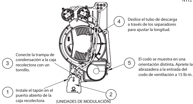
(UNIDADES DE MODULACIÓN) Configuración de la trampa horizontal a la derecha
